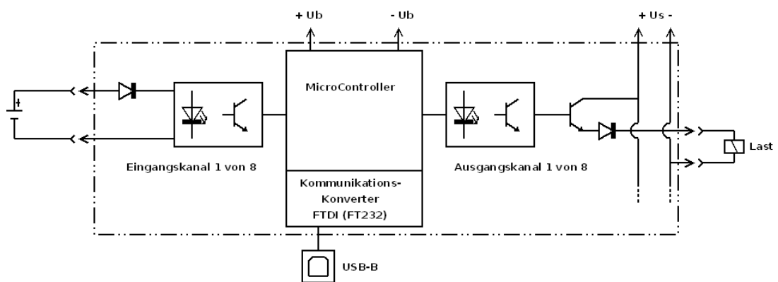
Prinzipschaltung
